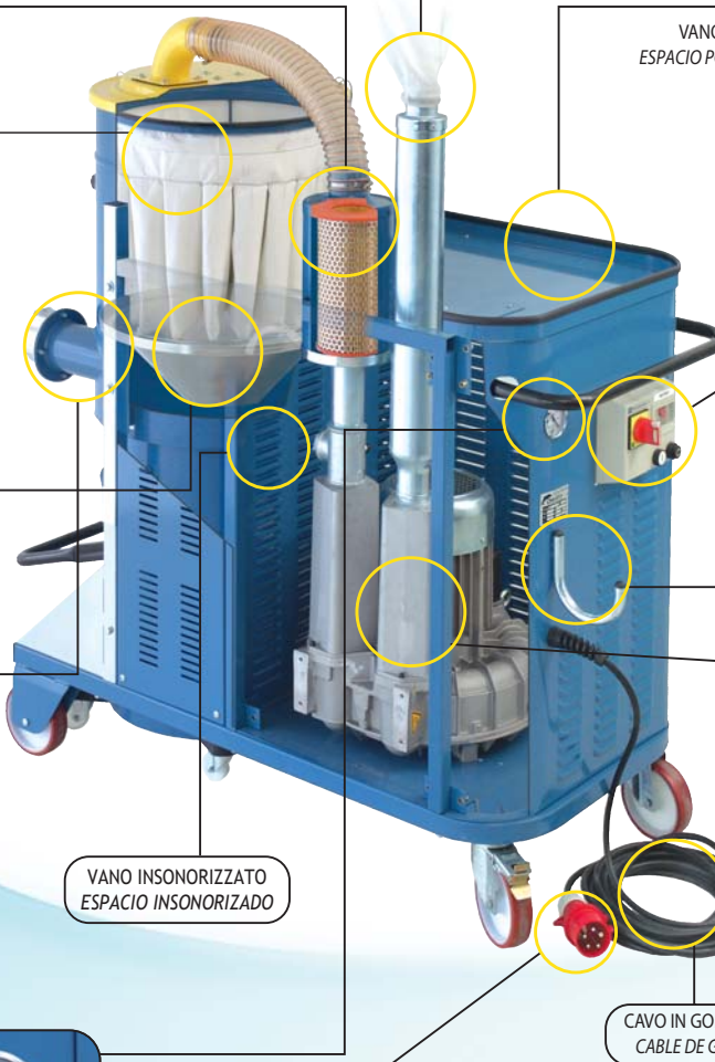
PREDISPOSIZIONE PER VALVOLA LIMITATRICE DI VUOTO PREDISPOSICIÓN PARA VÁLVULA LIMITADORA DE VACÍO
